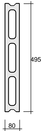
Doppio "mezzo blocco" (n. 10 pz per bancale)
